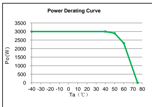
图3 R4850N6功率降额曲线
