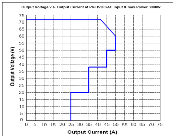
图1-1 输出外特性曲线（60V系统）
