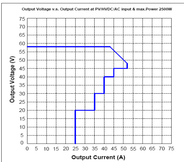
图1-2 输出外特性曲线（48V系统）
