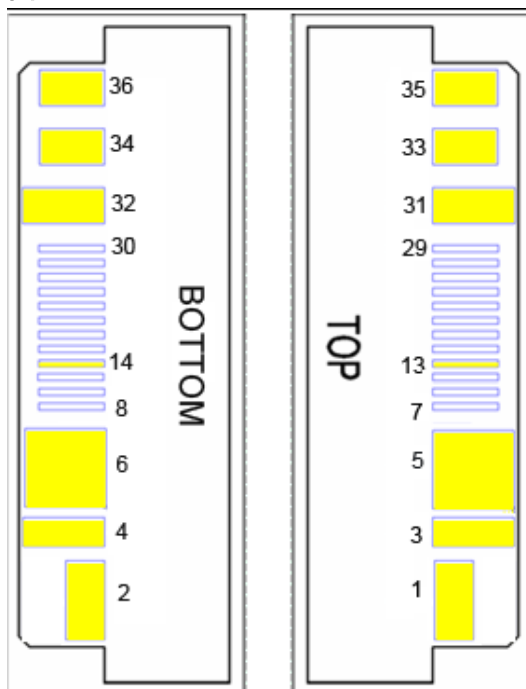
图1-6 模块金手指管脚示意图
