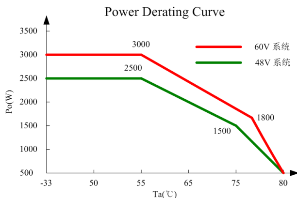
图1-3 功率高温降额曲线
