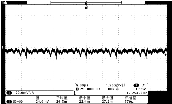
图 1. 输出电压纹波
