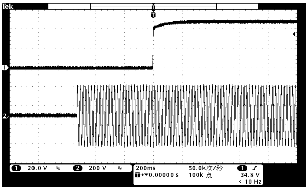
图 3. 启动波形
