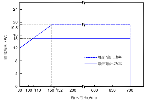
图2: 直流电压输入-输出功率降额曲线
