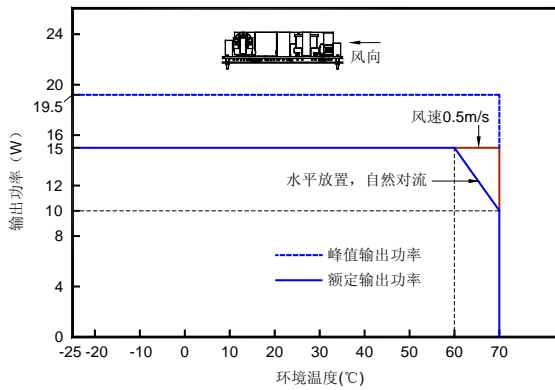
图3: 环境温度-输出功率降额曲线
